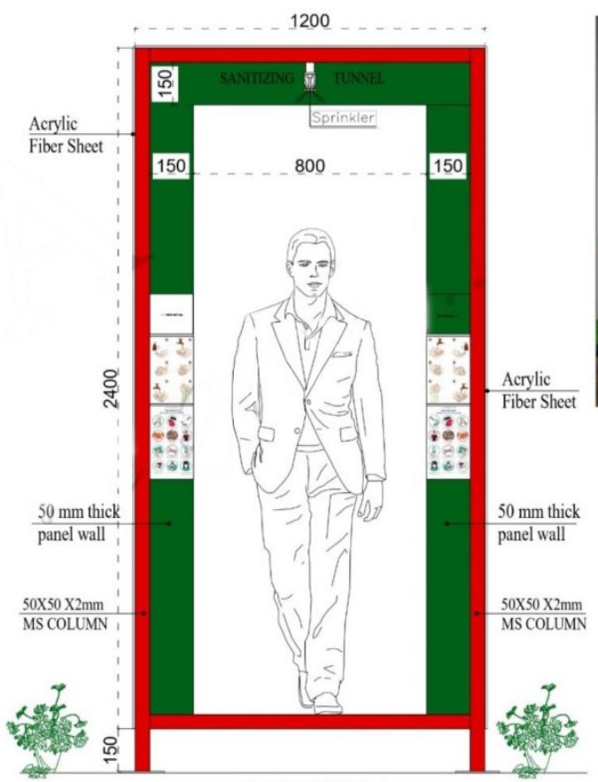
ELEVATION-A
